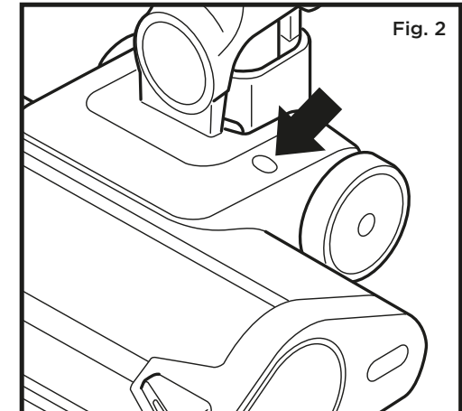
LIGHTDETECT-SENSOR
