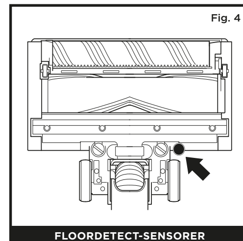
FLOORDETECT-SENSORER
