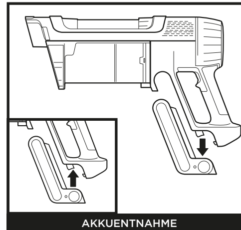
AKKUMENTNAHME
