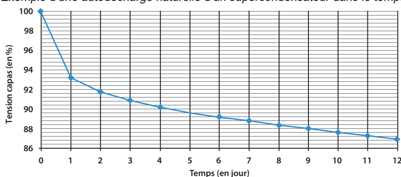
Exemple d'une autodécharge naturelle d'un supercondensateur dans le temps
