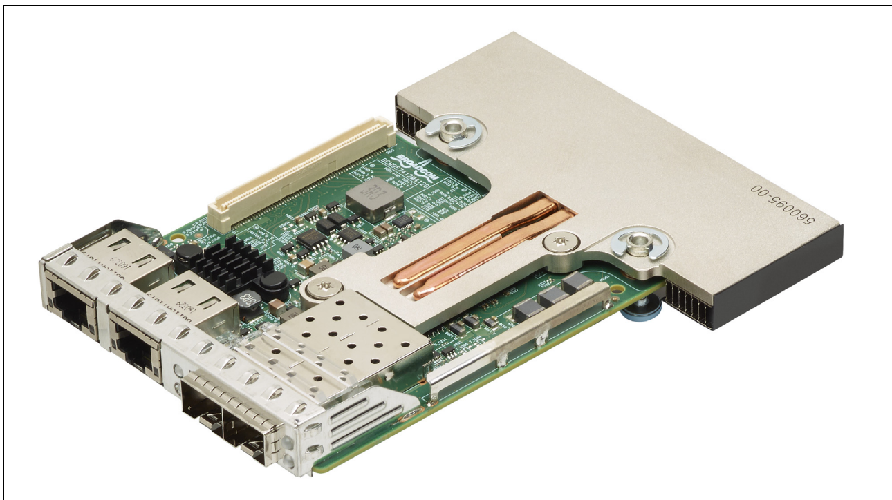
图 5: BCM957412M4120D 网络子卡 (rNDC)
