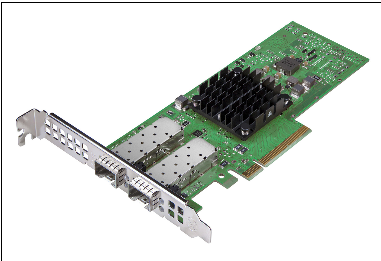
图 1: BCM957402A4020DC、BCM957412A4120D 网卡
