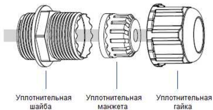
Рисунок 4: Водонепроницаемый уплотнитель для LAN-порта
