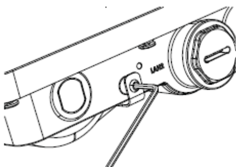
Рисунок 10: Затягивание крепежного винта
