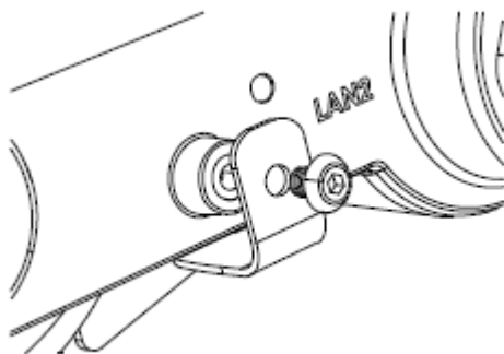
Рисунок 9: Установка крепежного винта
