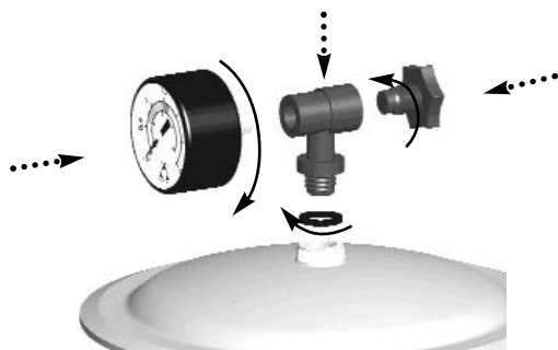
монтаж манометра при боковом вентиле
