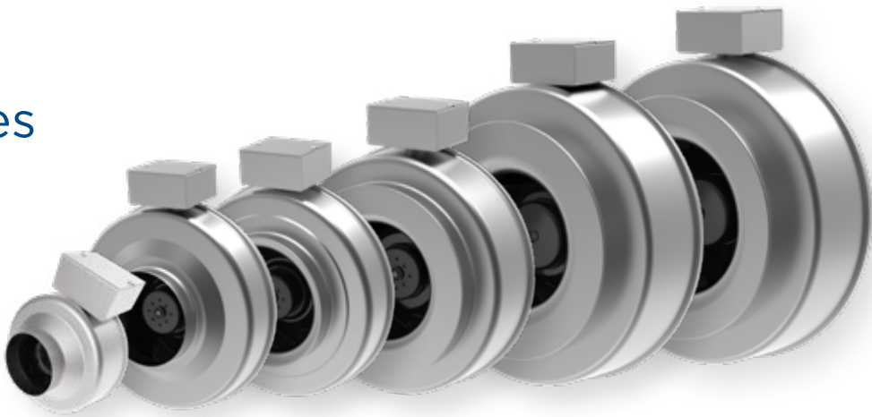
FG 4 XL EC FG 6M EC FG 8 EC FG 10 EC FG 12 EC FG 12XL EC
