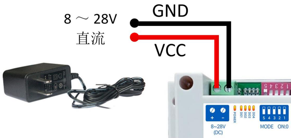
图 2-2-1 电源接线图
