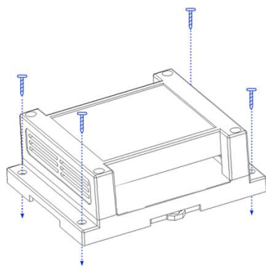
定位孔安装
