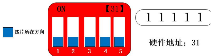
图 4-3-5 硬件地址 31
