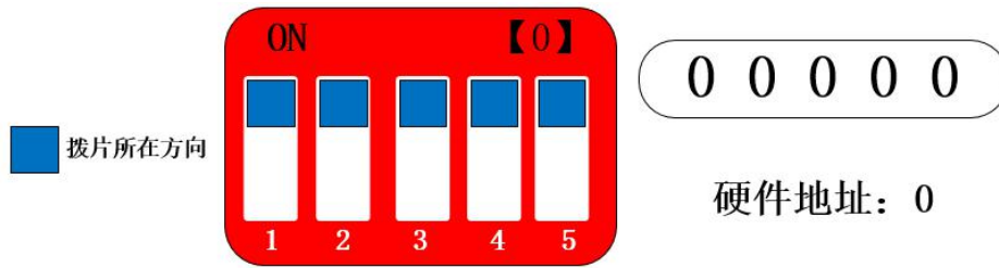
图 4-3-3 硬件地址 0
