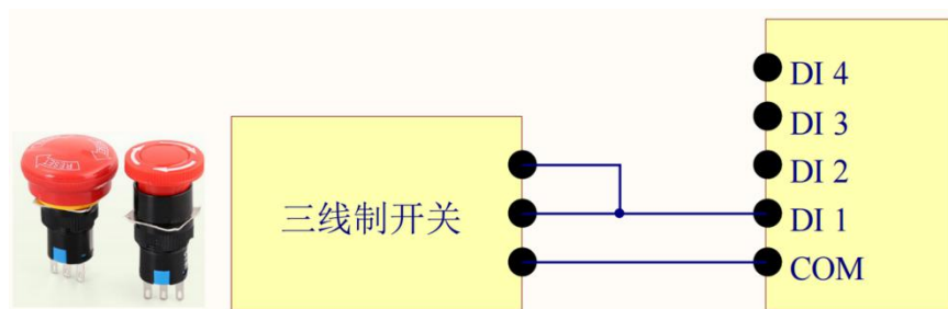
图 5-1-2 三线制开关接线图
