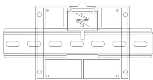
导轨安装
