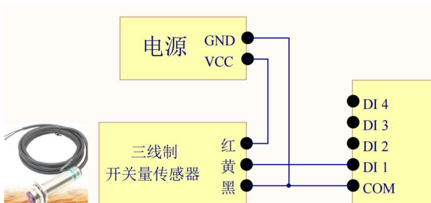
图 5-1-3 三线制传感器接线图
