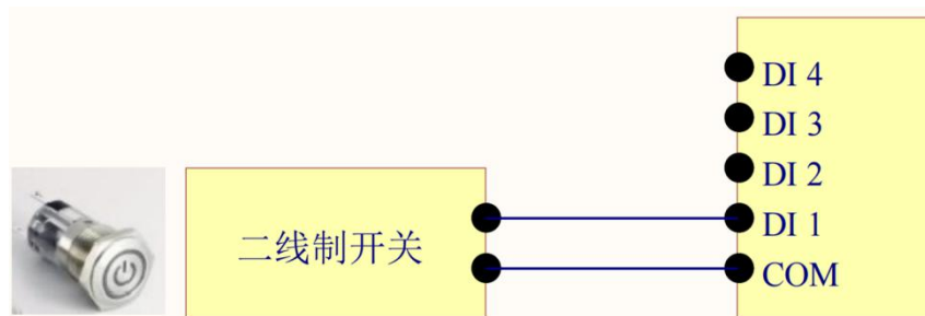
图 5-1-1 二线制开关接线图
