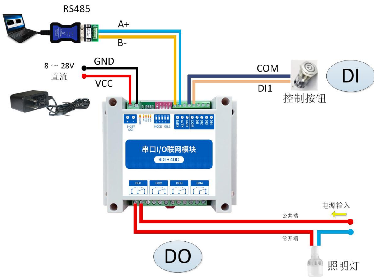
图 2-2-3 整体接线示意图
