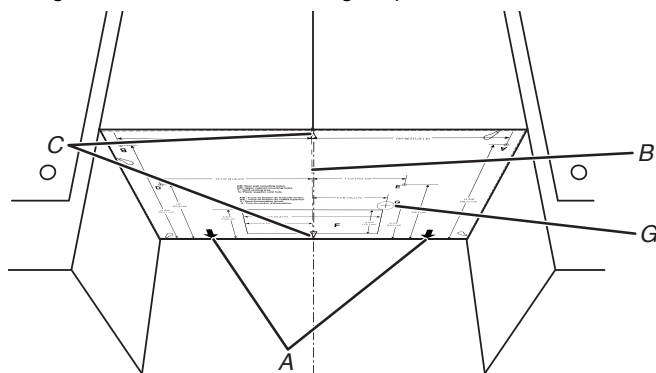
A. Flèches vers le mur B. Axe central de l'armoire supérieure C. Centrer les marques sur le gabarit en carton ou le gabarit pour l'armoire supérieure
