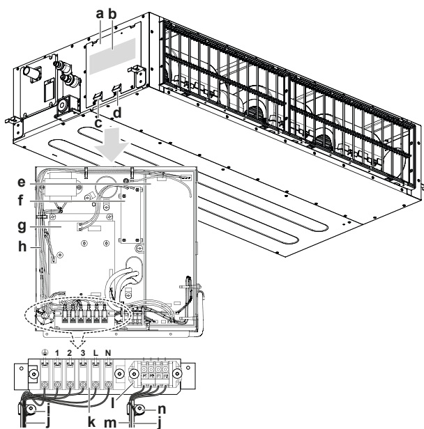
a Крышка распределительной коробки b Схема электропроводки c Порт для подключения кабеля силового электропитания d Порт для подключения проводов управления e Плата внутреннего блока 2 f Плата внутреннего блока 3 g Плата внутреннего блока 1 h Распределительная коробка i Пластмассовый хомут j Провод электропитания k Клеммы для подключения силового питания l Клеммы для подключения проводов управления
