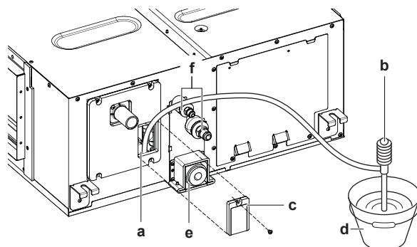
a Впуск воды b Переносной насос c Крышка отверстия для заливки воды d Емкость с водой (для заливки через отверстие) e Сливное отверстие для техобслуживания f Трубопровод хладагента
