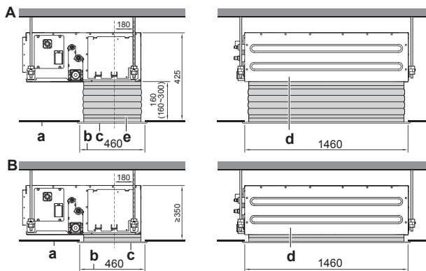
A Установка воздухозаборника с тканевым рукавом B Непосредственная установка воздухозаборной решетки a Поверхность подшивного потолка b Отверстие в подвесном потолке c Декоративная панель (дополнительное приспособление) d Внутренний блок (задняя сторона) e Тканевый рукав для соединения с декоративной панелью (дополнительное приспособление)
