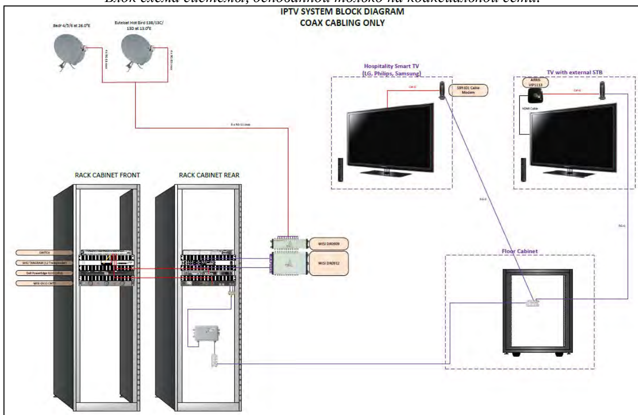
Блок схема системы, основанной только на коаксиальной сети.
