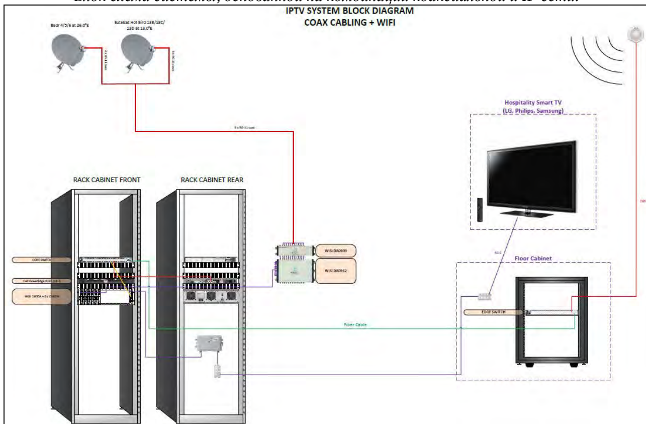
Блок-схема системы, основанной на комбинации коаксиальной и IP-сети.
