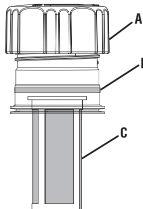
A - Bouchon de réservoir ventilé B - Ligne de remplissage maximale C - Filtre d'écran
