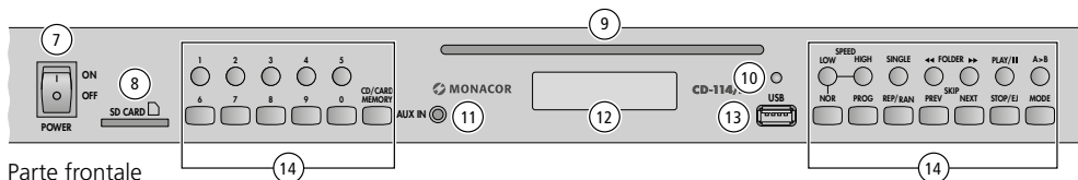
Parte frontale
