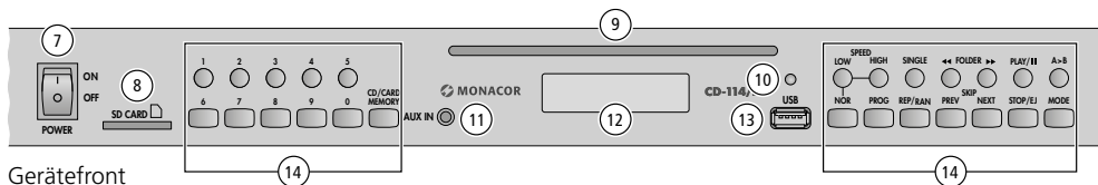
Gerätefront
