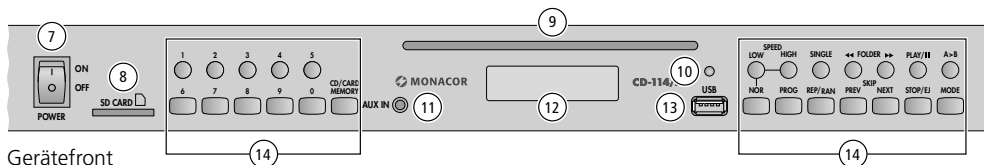
Gerätefront
