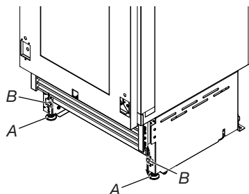
A. Pieds d'ajustement de l'aplomb B. Boulons de réglage
