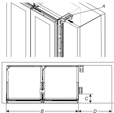
A. Bride antibascullement supérieure B. 35 1/2 po (901,7 mm) pour le modèle de 18 po et 47 9/16 po (1 208 mm) pour le modèle de 24 po C. 4 5/8 po (117 mm) D. 18 1/2 po (470 mm)
