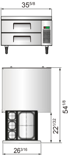
MGF8448GR
