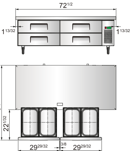
MGF8453GR
