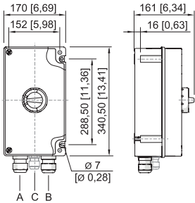
Esquema de medida (todas las medidas en [pulgadas]) – Se reserva el derecho a modificaciones
