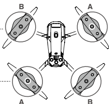
對準標記安裝螺旋槳
