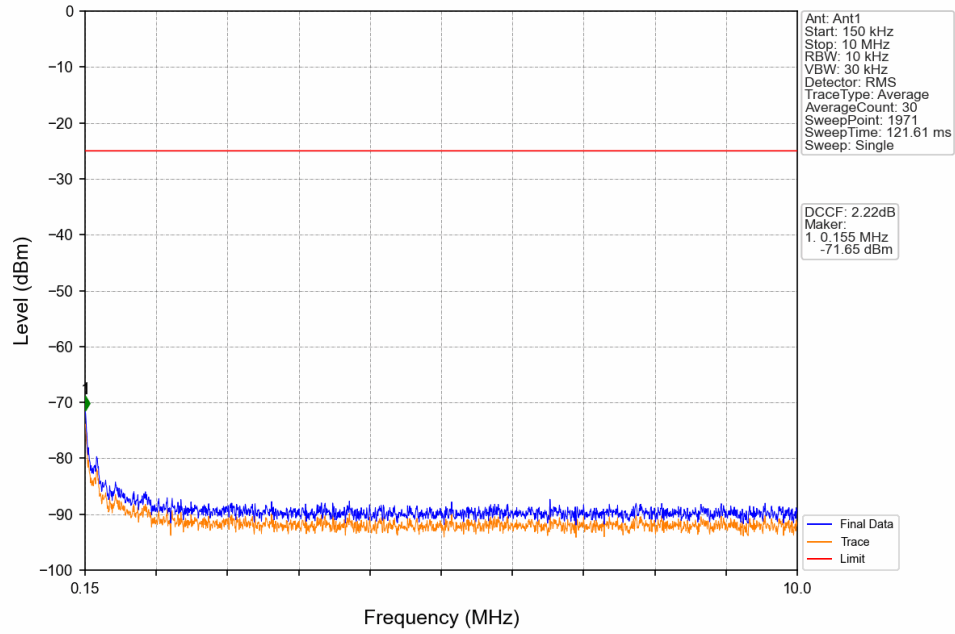
Band41_20MHz_QPSK_HCH_2680MHz_RB_1_99_NTNV
