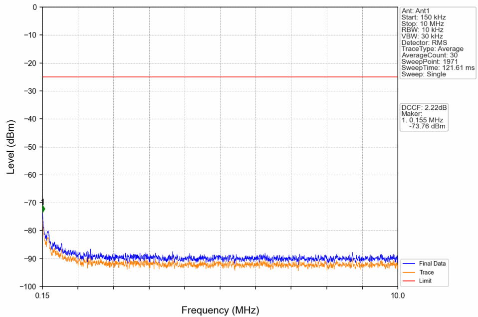
Band41_15MHz_QPSK_MCH_2593MHz_RB_1_0_NTNV
