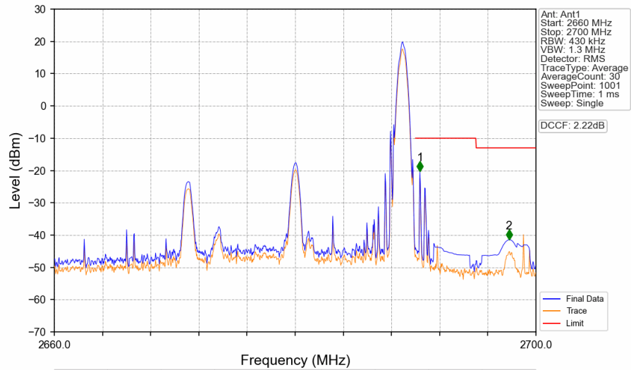
Band41_20MHz_QPSK_HCH_2680MHz_RB_1_99_NTNV
