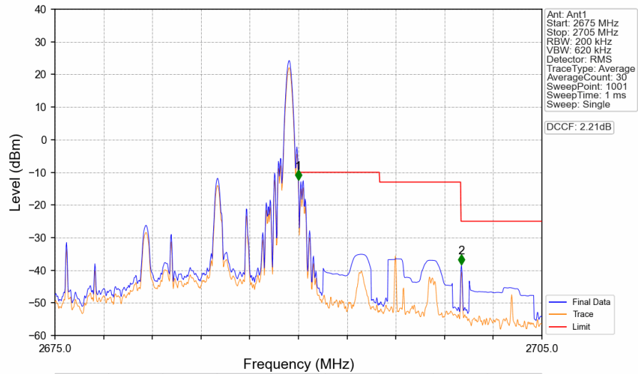
Band41_10MHz_QPSK_HCH_2685MHz_RB_1_49_NTNV
