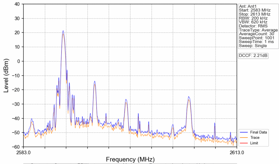
Band41_10MHz_16QAM_MCH_2593MHz_RB_1_0_NTNV
