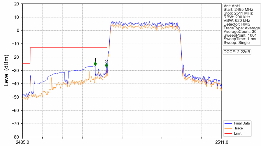
Band41_10MHz_16QAM_LCH_2501MHz_RB_50_0_NTNV
