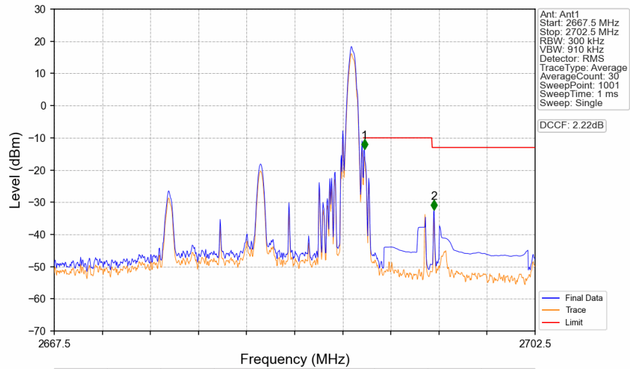
Band41_15MHz_QPSK_HCH_2682.5MHz_RB_1_74_NTNV
