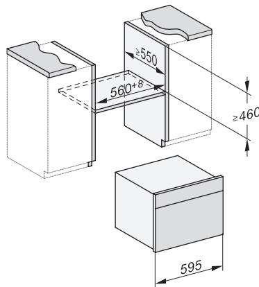
DGC7x4x, DGC7x4xX Skizze
