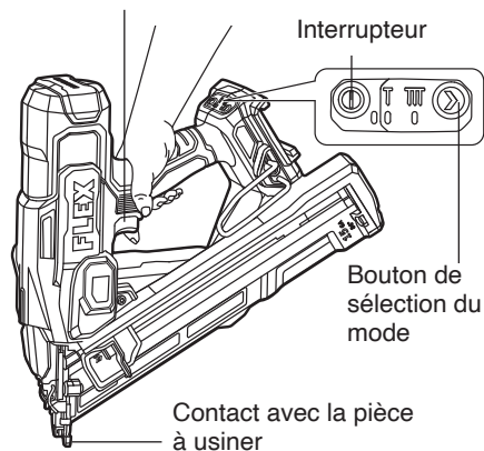
Fig. 7 Interrupteur à gâchette
