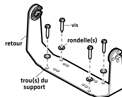
Installation du support à cardan
