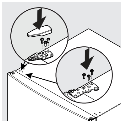
Top Hinge
