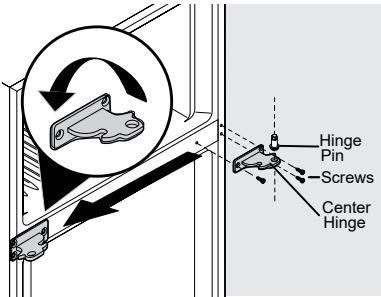
Center Hinge
