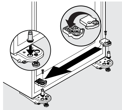
Door Stopper
