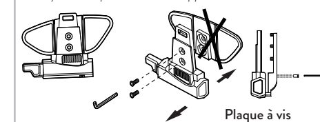
Plaque à vis
