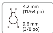
Orifice à l'arrière de l'enceinte
