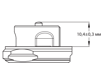
Розміри в закритому положенні для DN 15-32
