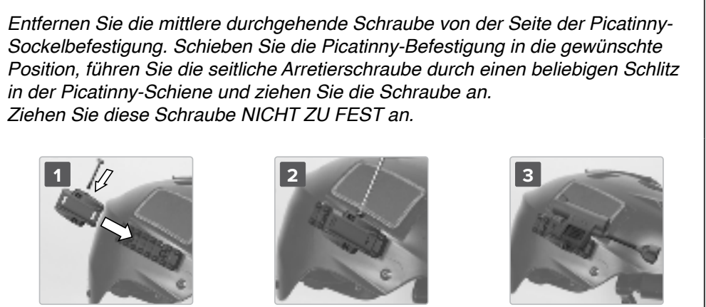
Abbildung 8 – Picatinny-Schienenbefestigung
