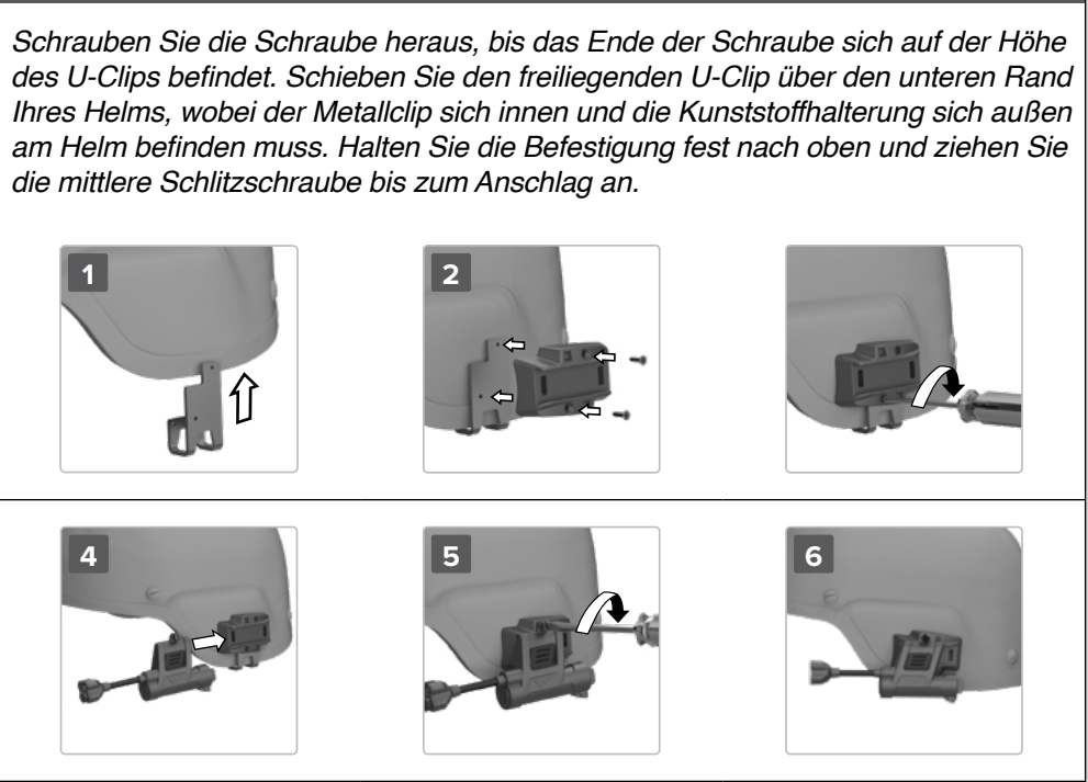
Abbildung 7 – Installation der MICH-Befestigung
