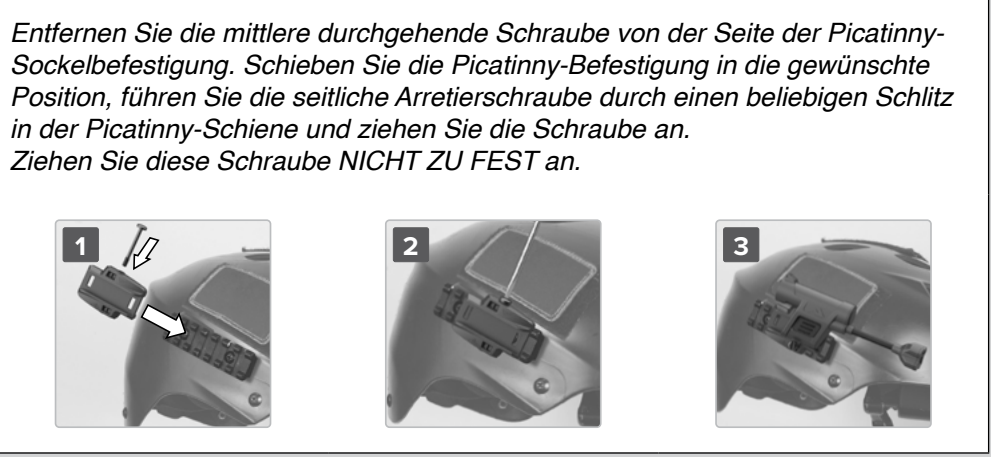
Abbildung 8 – Picatinny-Schienenbefestigung
