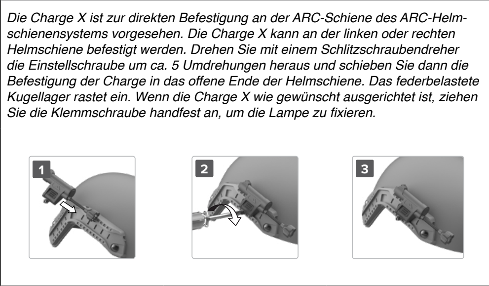
Abbildung 4 – Installation der ARC-Schiene
