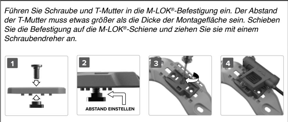
Abbildung 6 – M-LOK®-Befestigung
