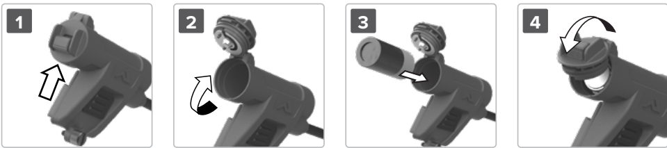
Figura 1 – Colocación de la batería
