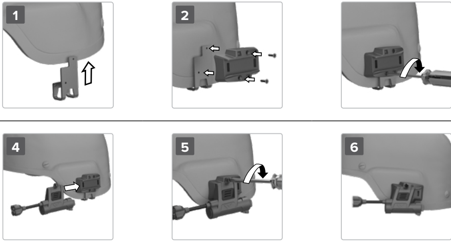
Figura 8 – Montaje en riel Picatinny
