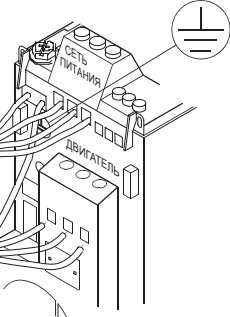
Рис. 1. Подключение заземляющего кабеля, проводов сети и двигателя
