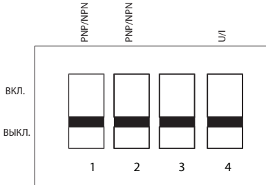
Рис. 3. Переключатели S200, 1–4
