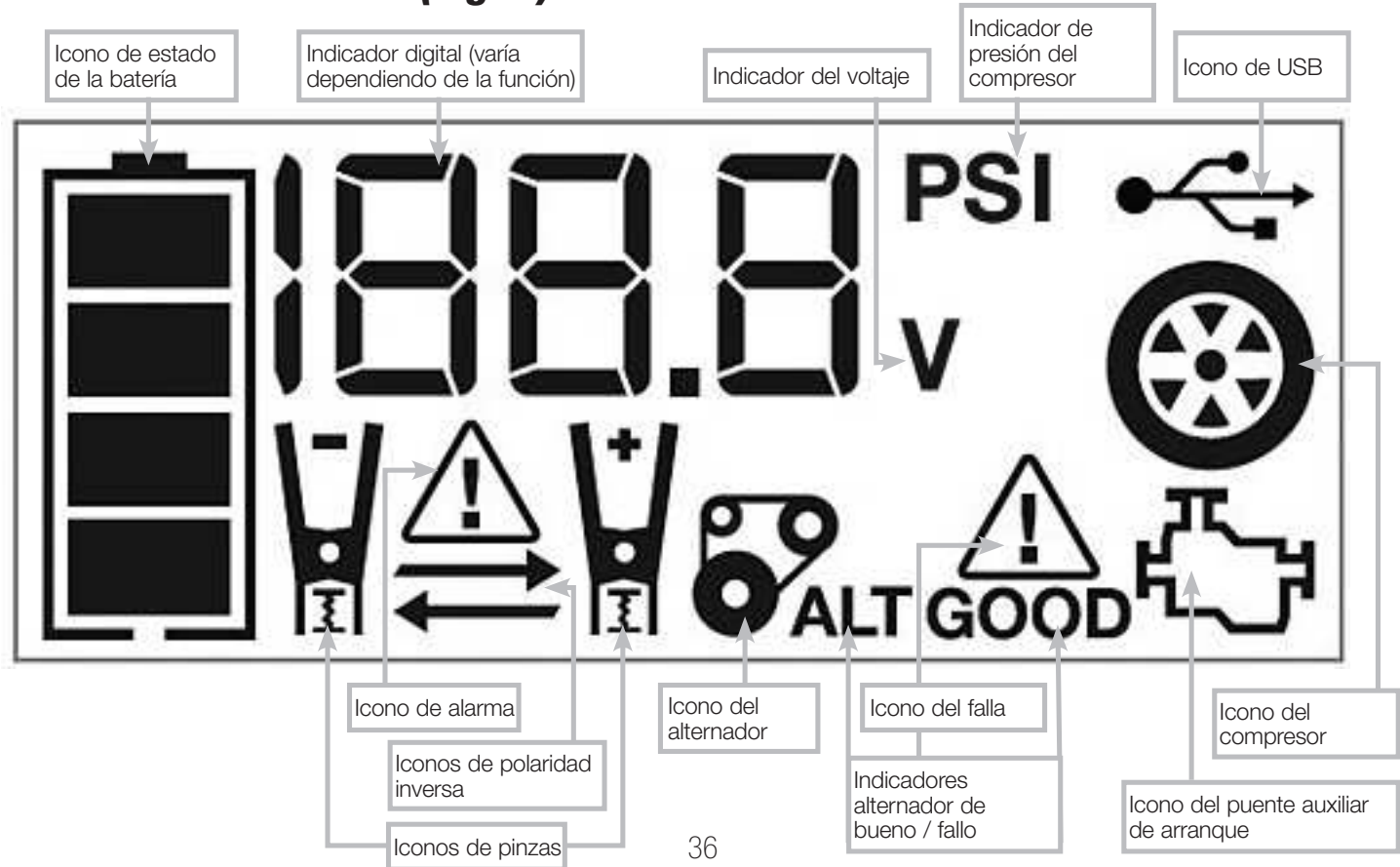
Pantalla LCD detalles (Fig. 3)
