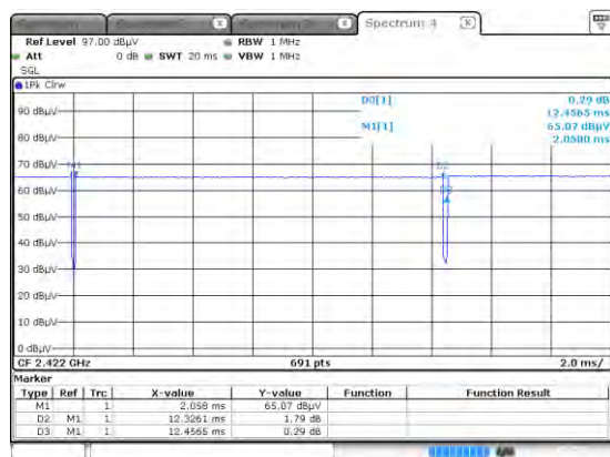
802.11b:
