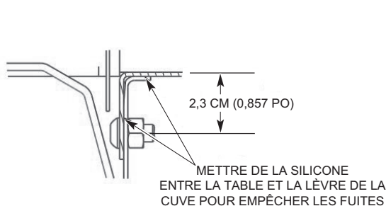
VUE EN COUPE DU RACCORDEMENT DE LA TABLE
