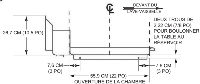
VUE DE L'EMPLACEMENT DES TROUS DANS LA SECTION DE LA TABLE TOURNÉE VERS LE BAS
