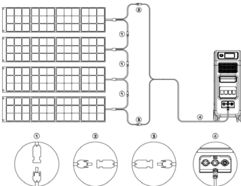
(A napelemből töltés lépései )
