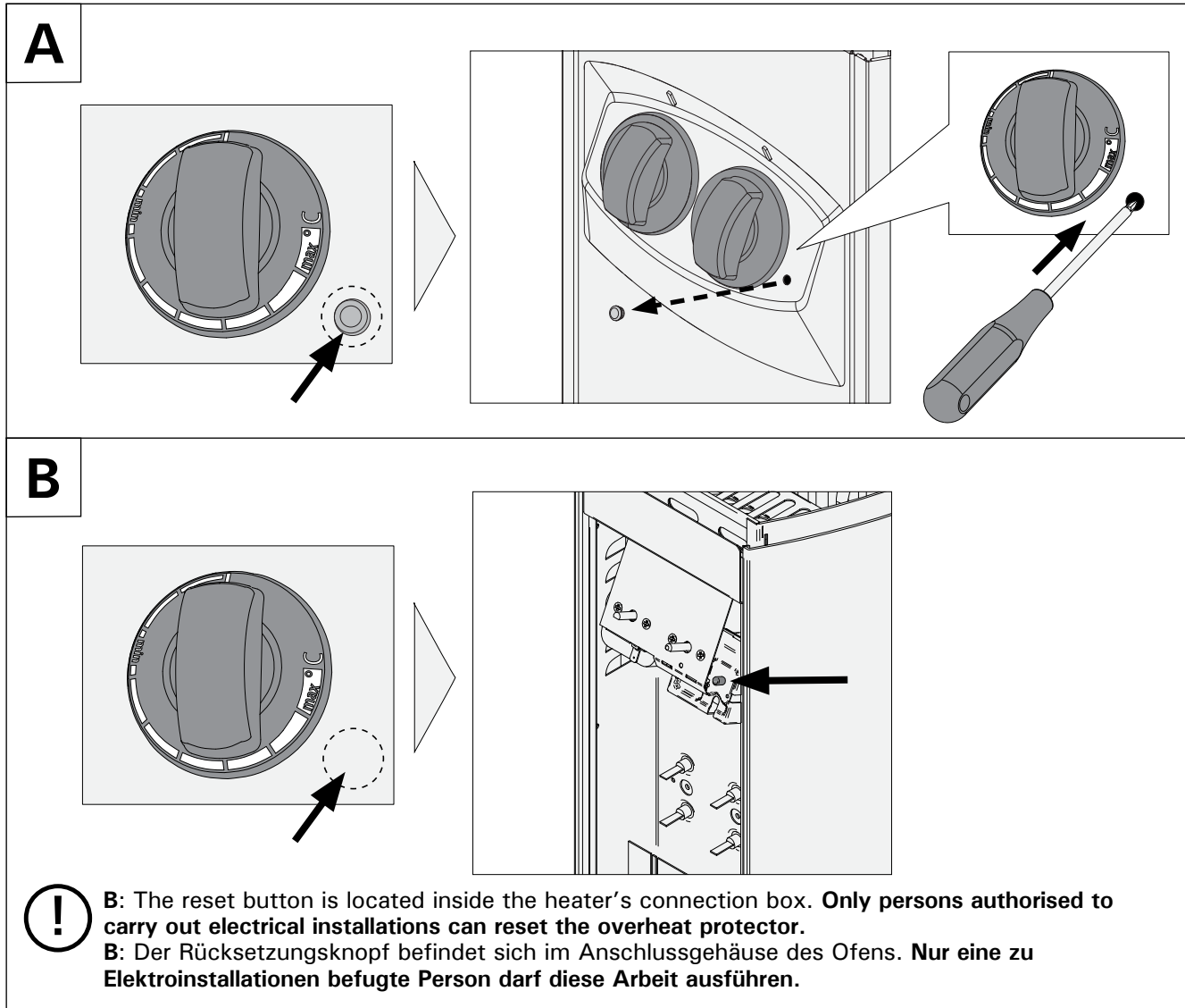
Figure 9. Reset button for overheat protector Abbildung 9. Rücksetzkнопf des Überhitzungsschutzes
