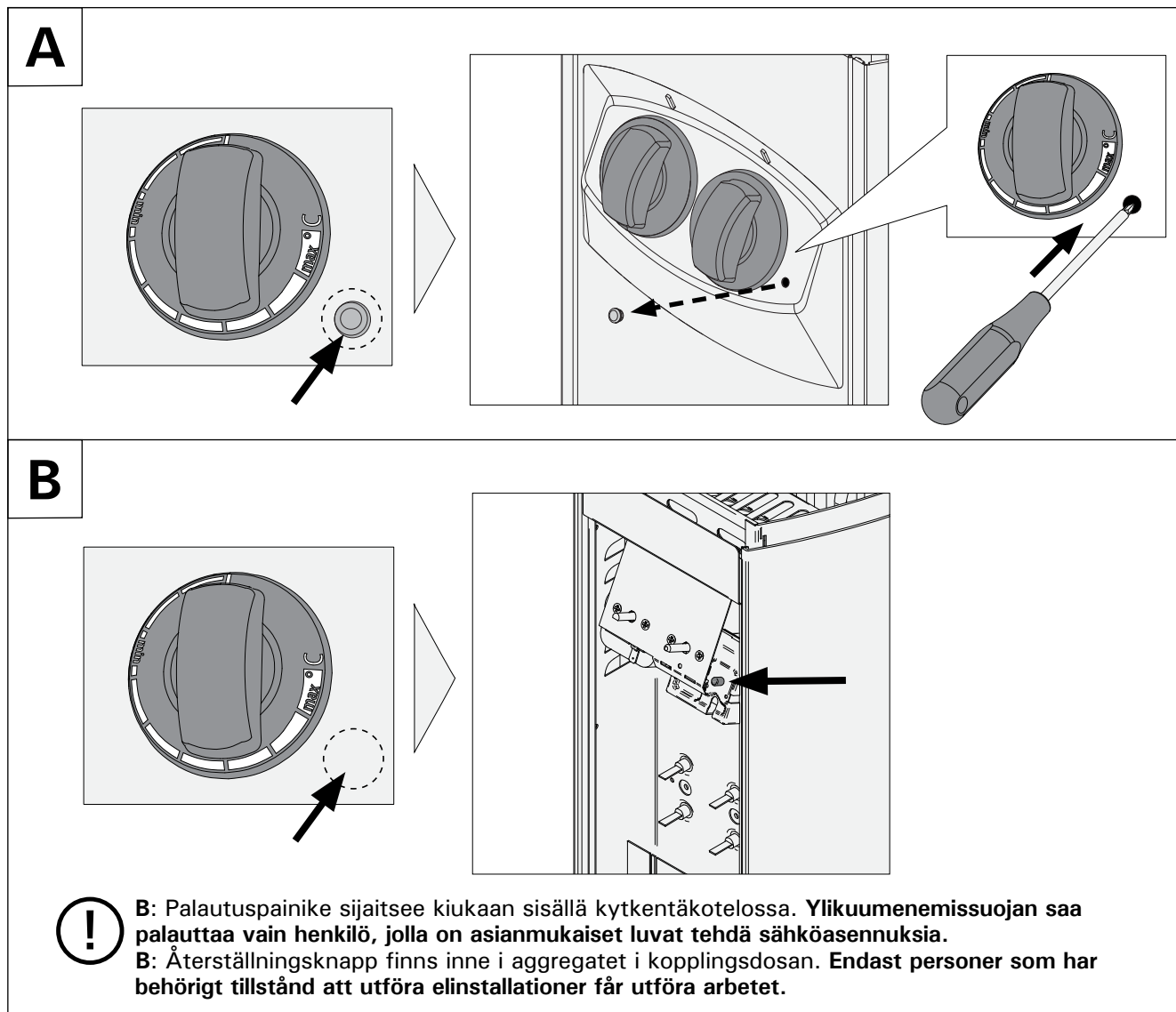
Kuva 9. Ylikuumenemissuojan palautuspainike
