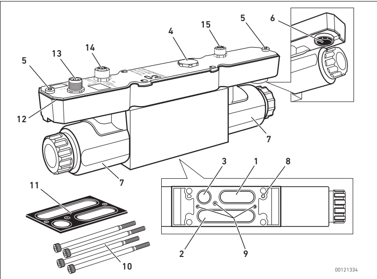
Abb. 1: ED07-Druckregelventil
