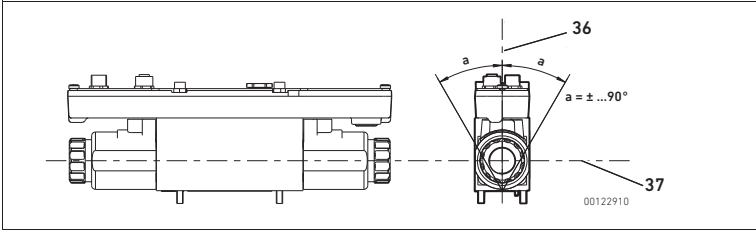
fig 3: Monteringsläge
