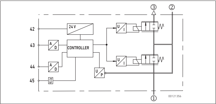
fig 4: Funktionsplan
