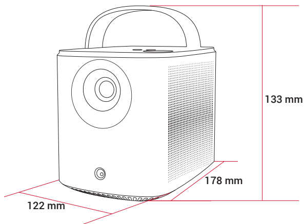
尺寸
