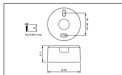
OccuSwitch LRM1070 opbouwdoos afmetingen in mm
