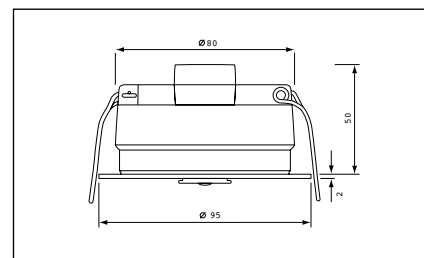
OccuSwitch LRM1070 afmetingen in mm
