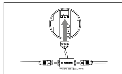
Wieland aansluitkabel LCC1070
