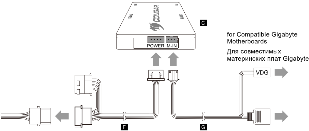
Molex 4 pin Connector of the Power Supply Cables Коннектор питания Molex 4 pin
