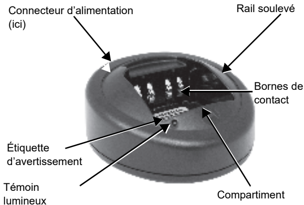
Figure 1 : Chargeur de batteries
