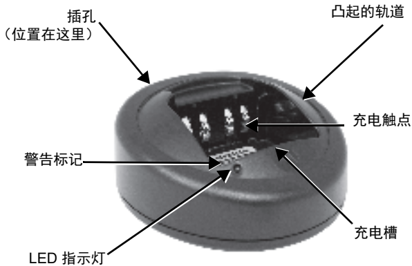
图 1: 电池充电器
