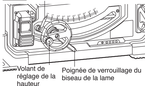
Fig. 24 Indicateur
