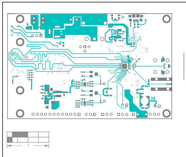
MAX96717 EV Kit—Top
