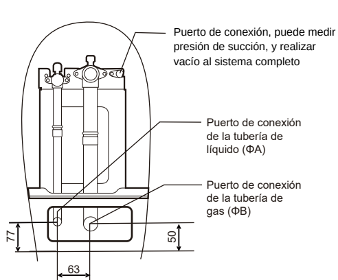
Figura 8 Detalle R1, R2
