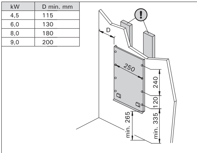
9. ábra A fali szerelvény elhelyezése (a méretek milliméterben értendők)
