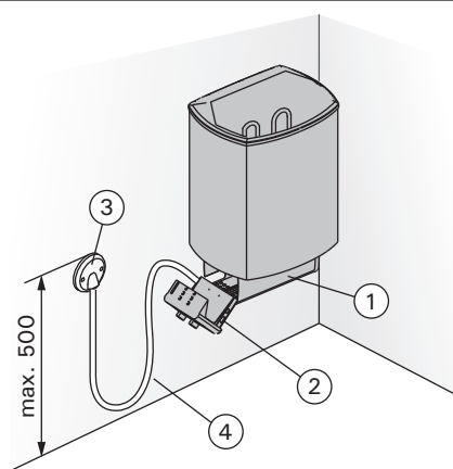
Figure 10. Raccord du poêle Figuur 10. Verbindingen van de kachel
