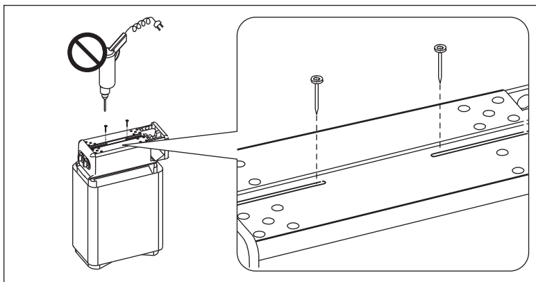
Figura 7. Remoção dos parafusos de aperto da extremidade
