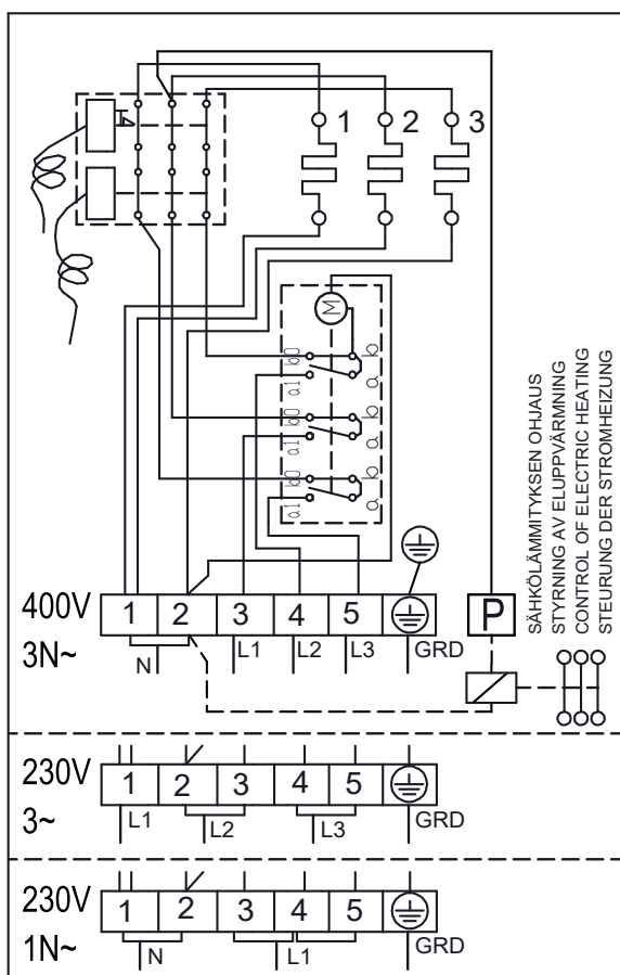
Figura 13. Conexiones eléctricas (1)
