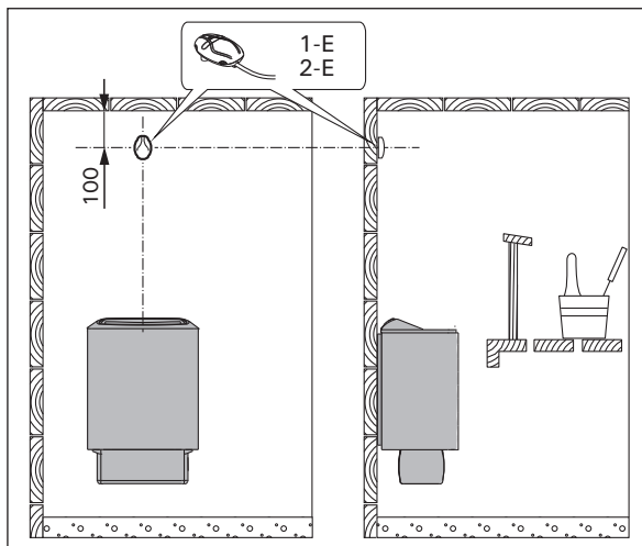
Figura 11. nstalación del sensor (todas las dimensiones en milímetros)
