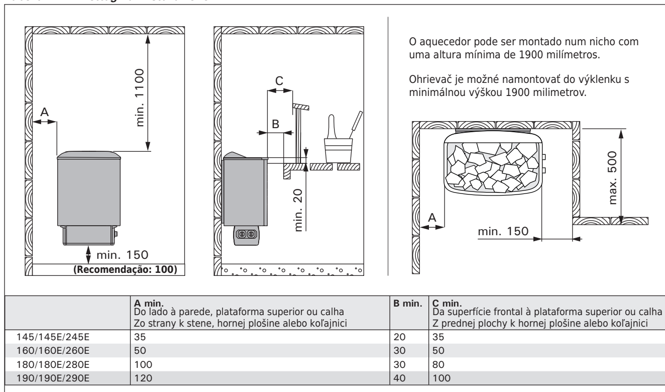
Figura 6. Distancias de seguridad (todas las dimensiones en milímetros)
