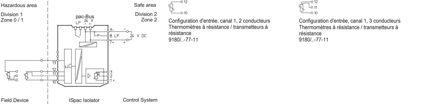
Schéma de raccordement 9180/1.-77-11
