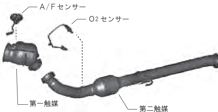
純正触媒構成図
