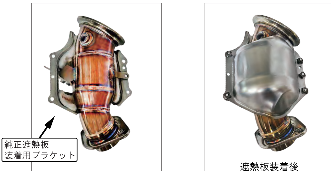
図4. 純正遮熱板取付け参考図
