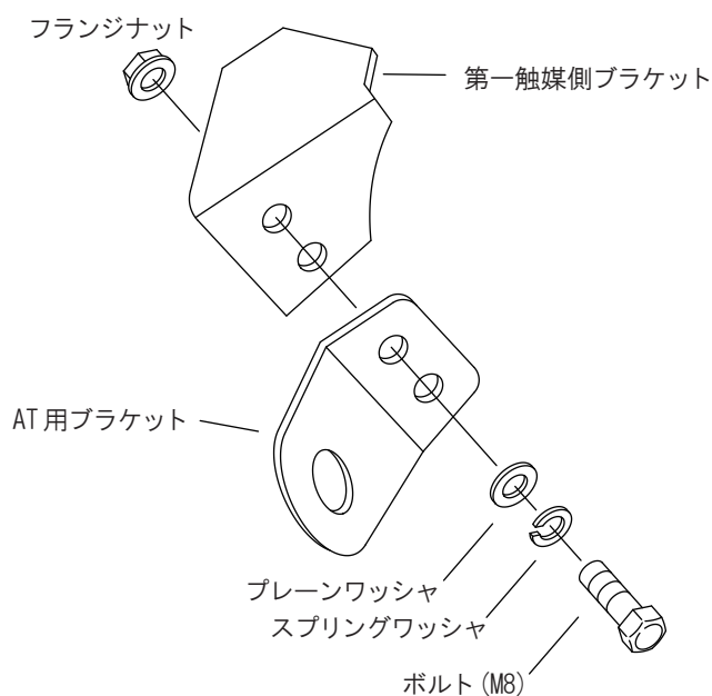
図3. AT 車用ブラケット組付け図
