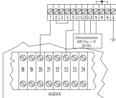
Configurazione Resistenza integrativa 4kW alimentata a 400 Vac + N 50 Hz
