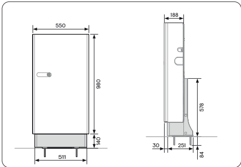
Montage au sol avec socle (vendu séparément)
