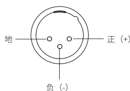
端口极性示意
