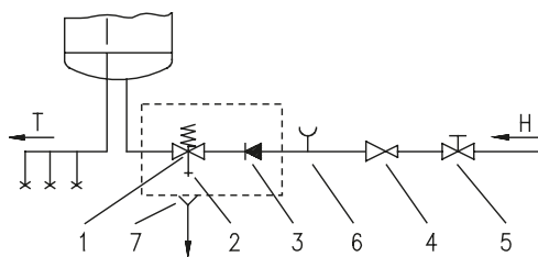
Das Drucksystem
