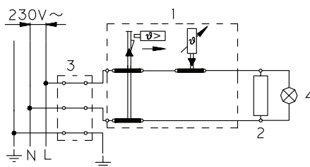
Schéma elektrické přípojky
