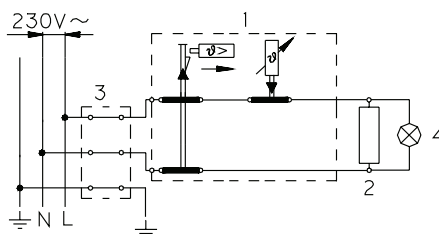
Электросхема
