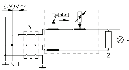
Schema van de elektrische verbinding
