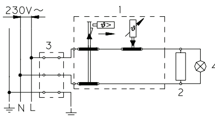
Az elektromos kapcsolás vázlata
