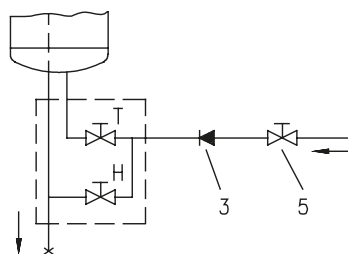
Das Durchflußsystem
