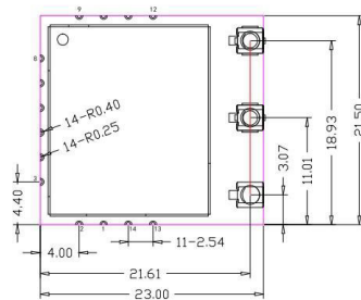
模组俯视图
