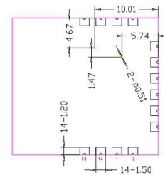
模组底视图
