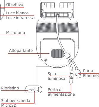
Vista posteriore
