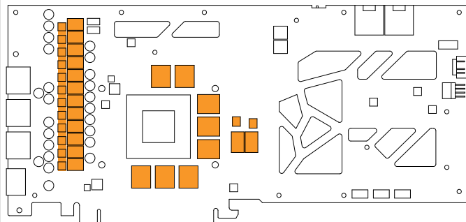
Thermal Pad F 1.0mm
